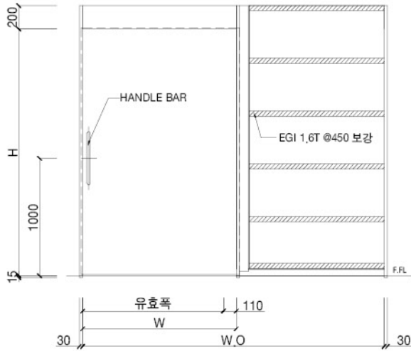
ELEVATION
